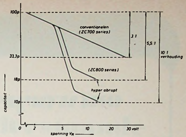
Fig. 8. Conventionele en hyper abrupte afstemdioden.
